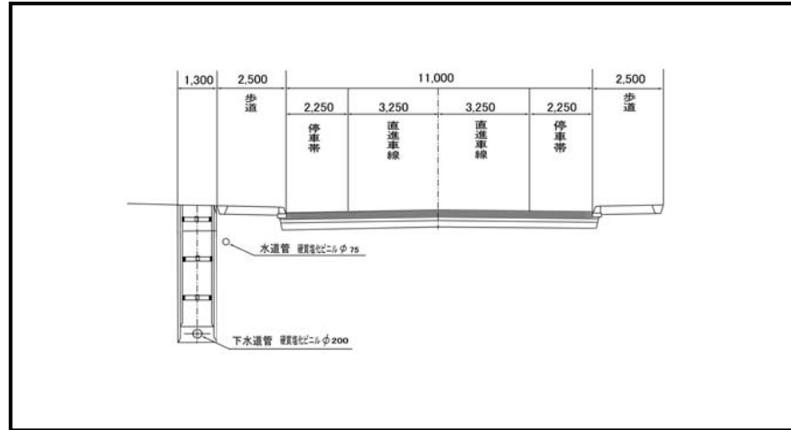
標準土工定規図
